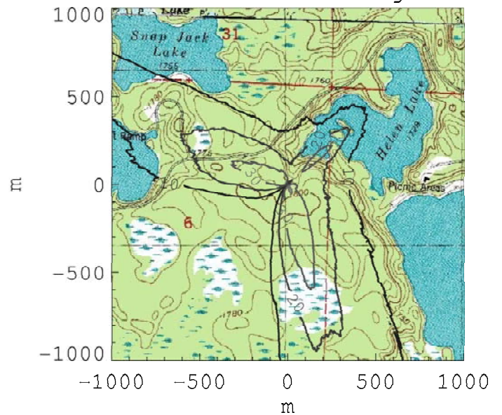
Summer nonSW Night
